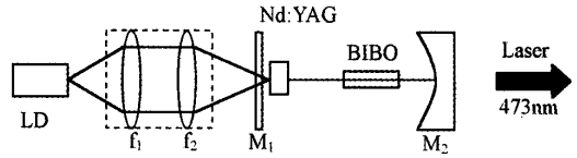
图 1 实验装置图 Fig. 1 Experiment setup
