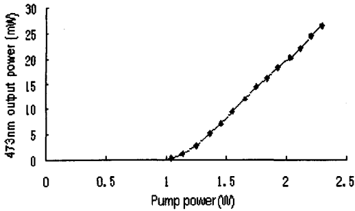
图2 蓝光输出随泵浦功率的变化曲线
